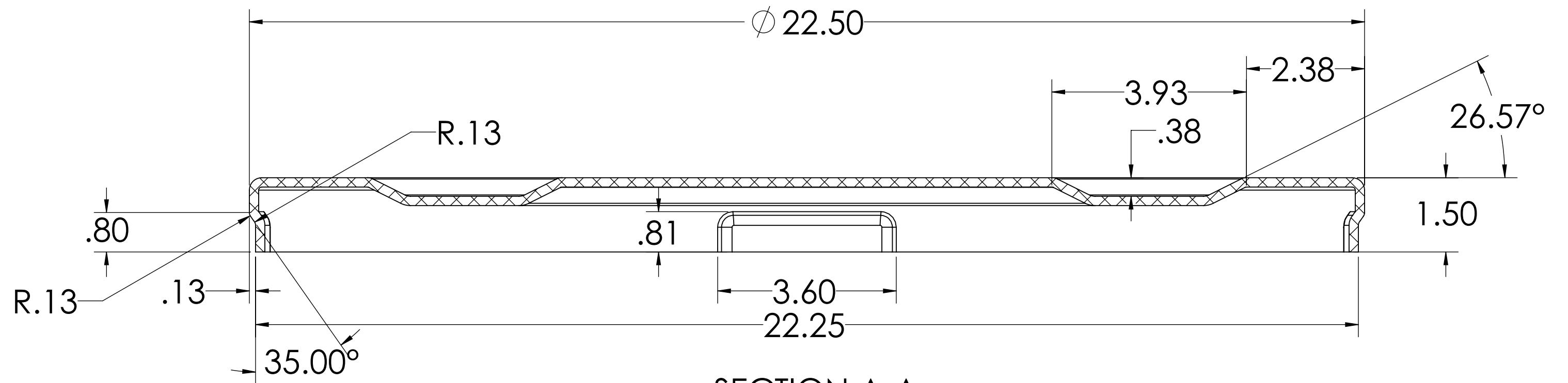
SECTION A-A SCALE 1 : 2
