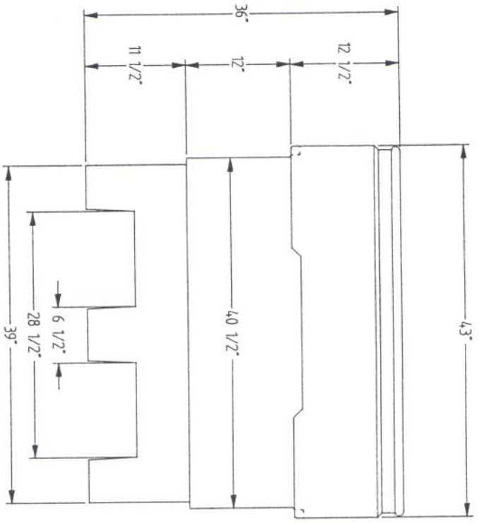
END ELEVATION
