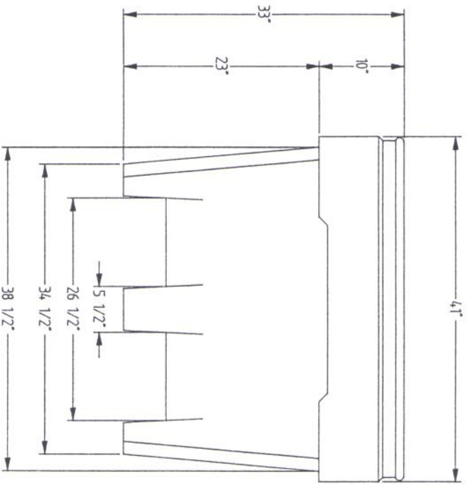
END ELEVATION
