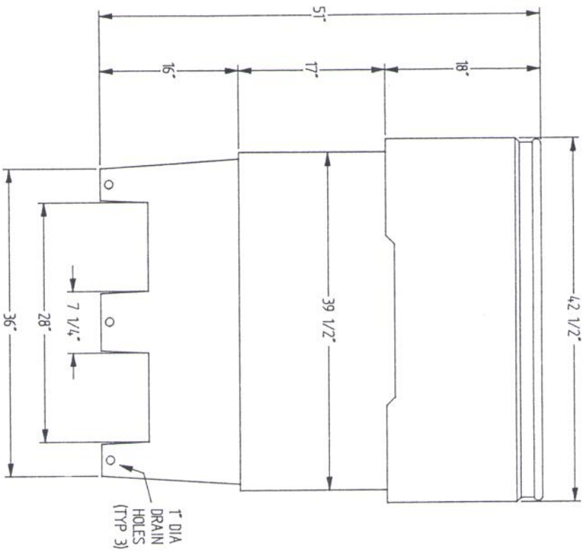
END ELEVATION
