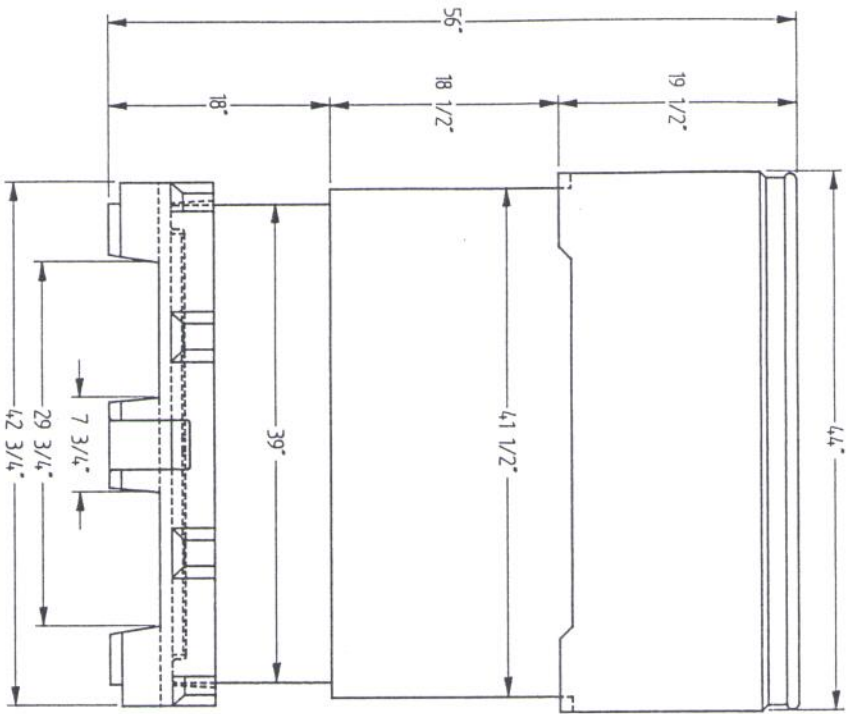
END ELEVATION
