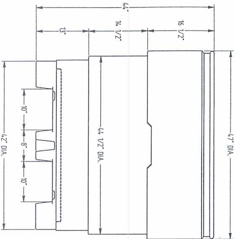
END ELEVATION
